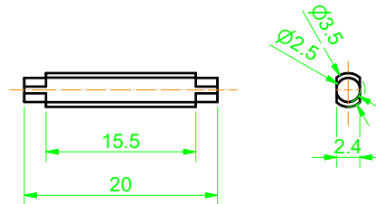
連桿軸2X8
