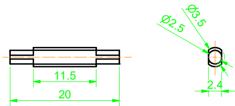
連桿軸3X16
