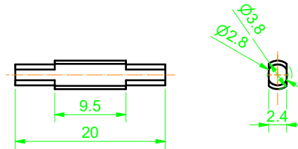
連桿軸4X8
