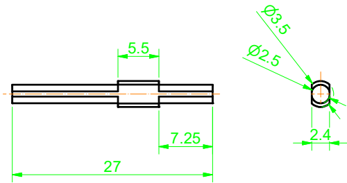
連桿軸1X8
