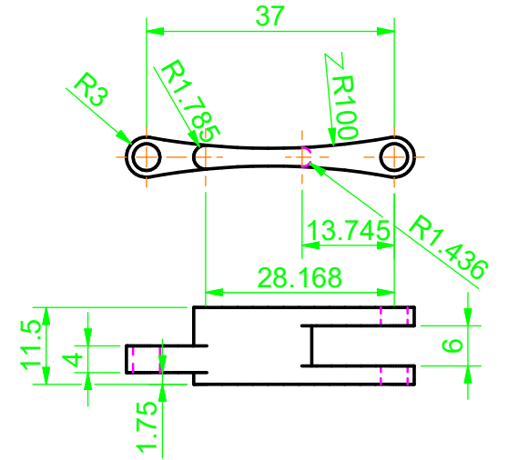
連桿4X8
