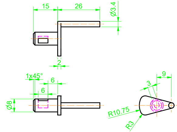
偏心軸X4
