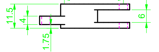
連桿4X8
