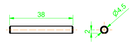
連桿軸5X4
